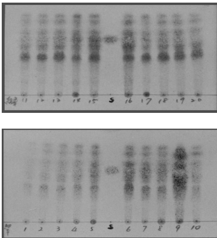
圖 1 細辛的 TLC 圖
