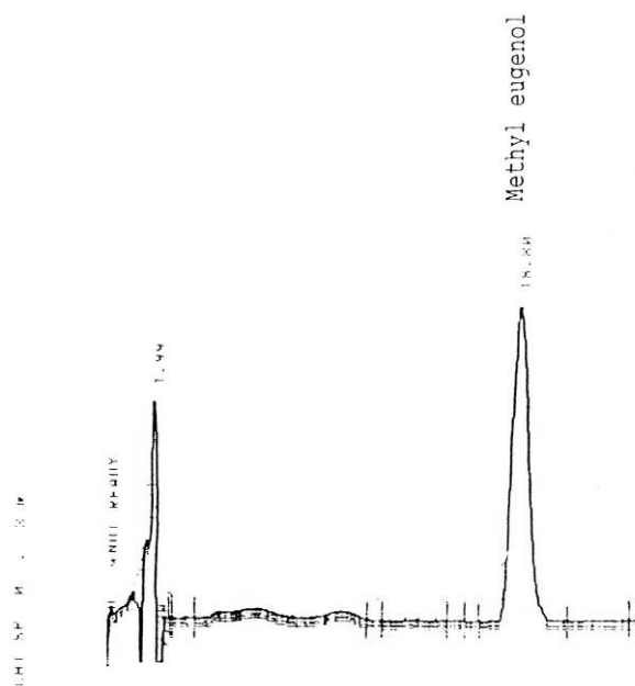
圖 2 細辛的指標成分之 HPLC 圖
