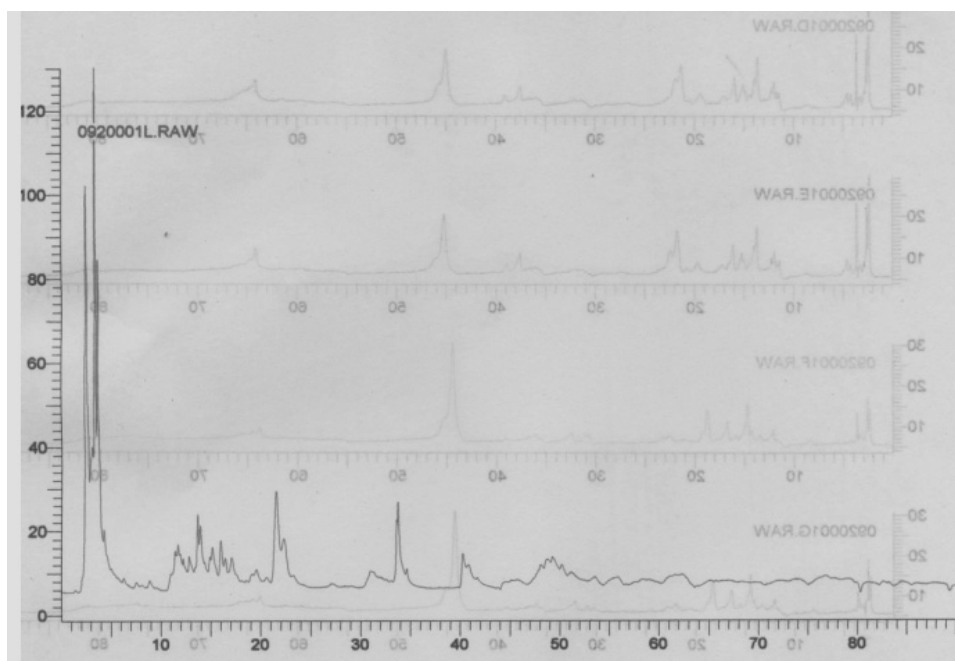
圖 D01-54-3b 沙苑蒺藜（中部）甲醇萃取之 HPLC 圖
