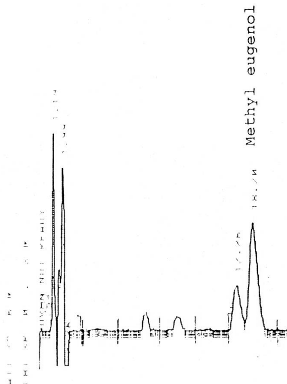
圖 3 細辛的 HPLC 圖
