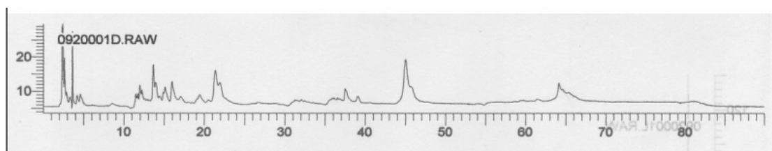
圖 D01-54-3a 沙苑蒺藜（北部）甲醇萃取之 HPLC 圖
