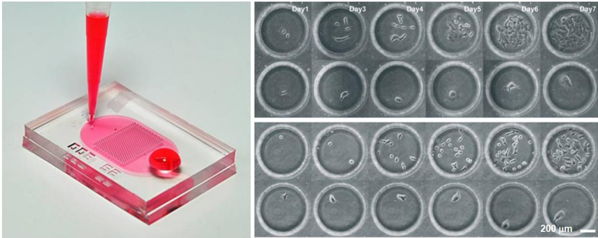
【圖片說明】微流體雙微井單細胞培養晶片及細胞培養過程
